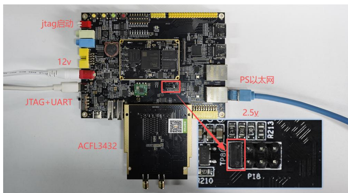
图 1-28 硬件连接图
