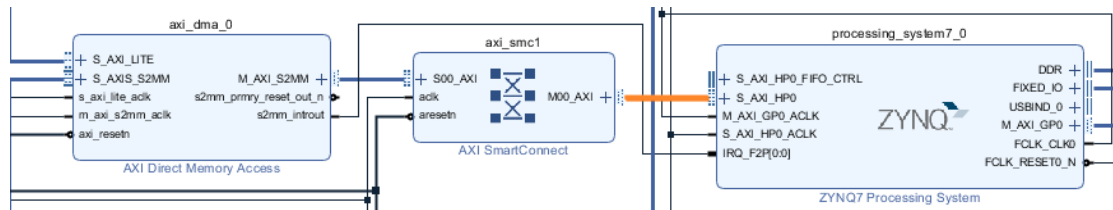
图 1-19 DMA 模块和 AXI HP0 接口连接
