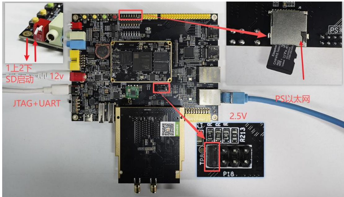
图 1-2 硬件连接图
