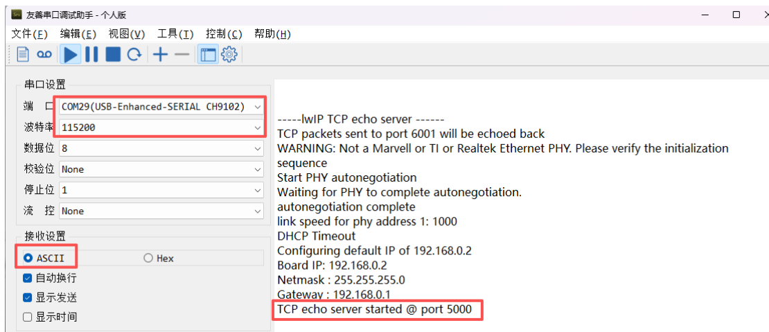
图 1-3 串口调试助手界面
