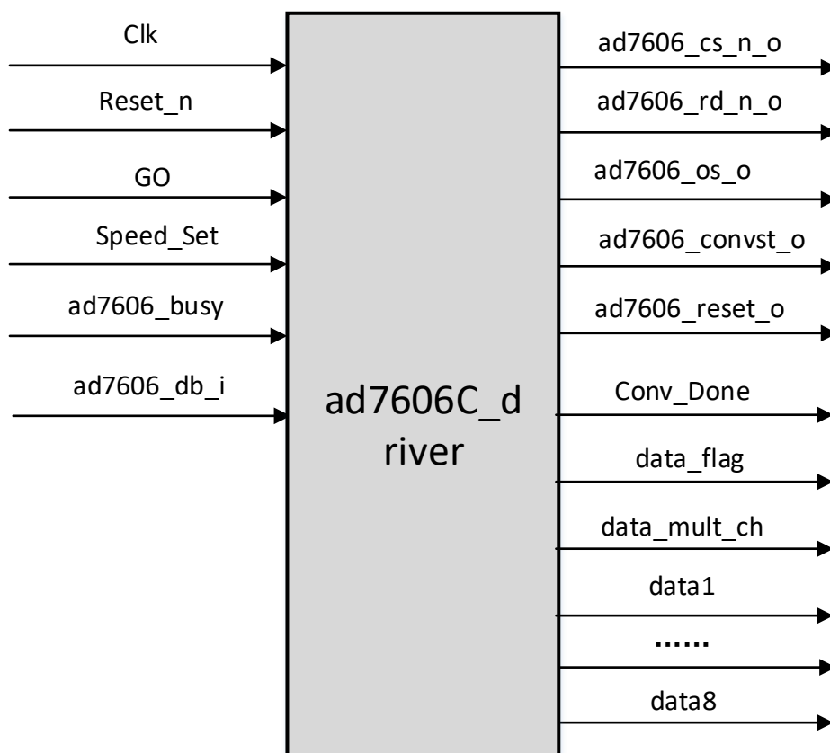
图 1-17 AD7606C 控制器驱动模块结构框图
