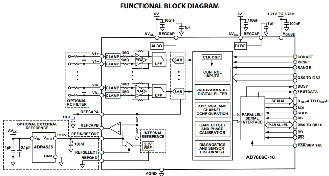
图 1-2 AD7606C 功能框图
