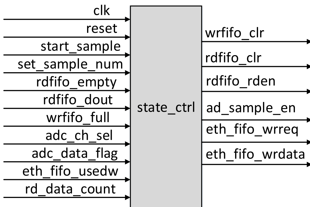
图 1-18 state_ctrl 模块结构框图
