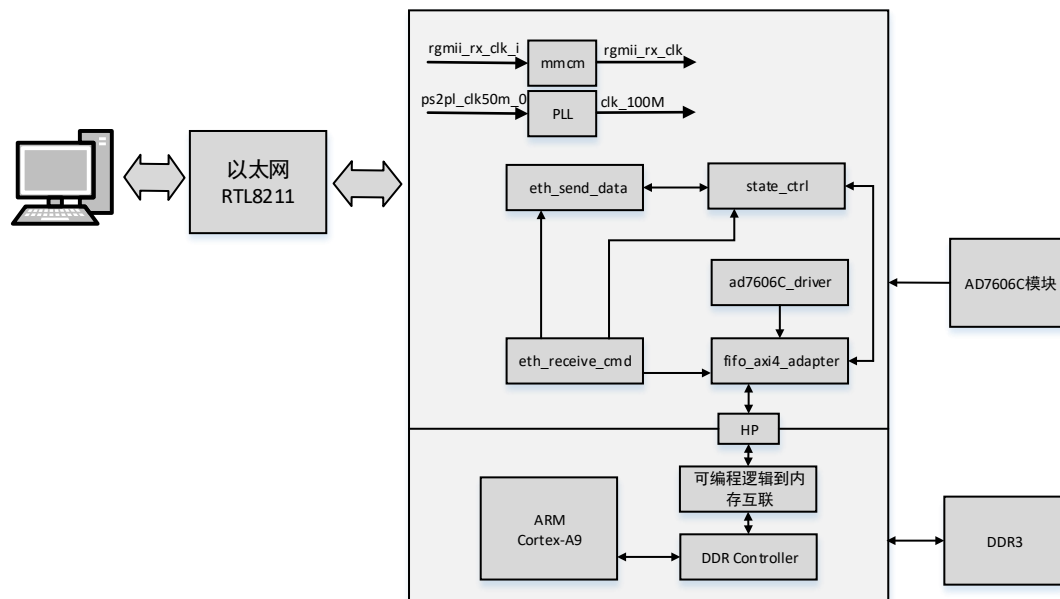
图 1-13 千兆以太网传输 AD7606C 数据采集整体设计框图
