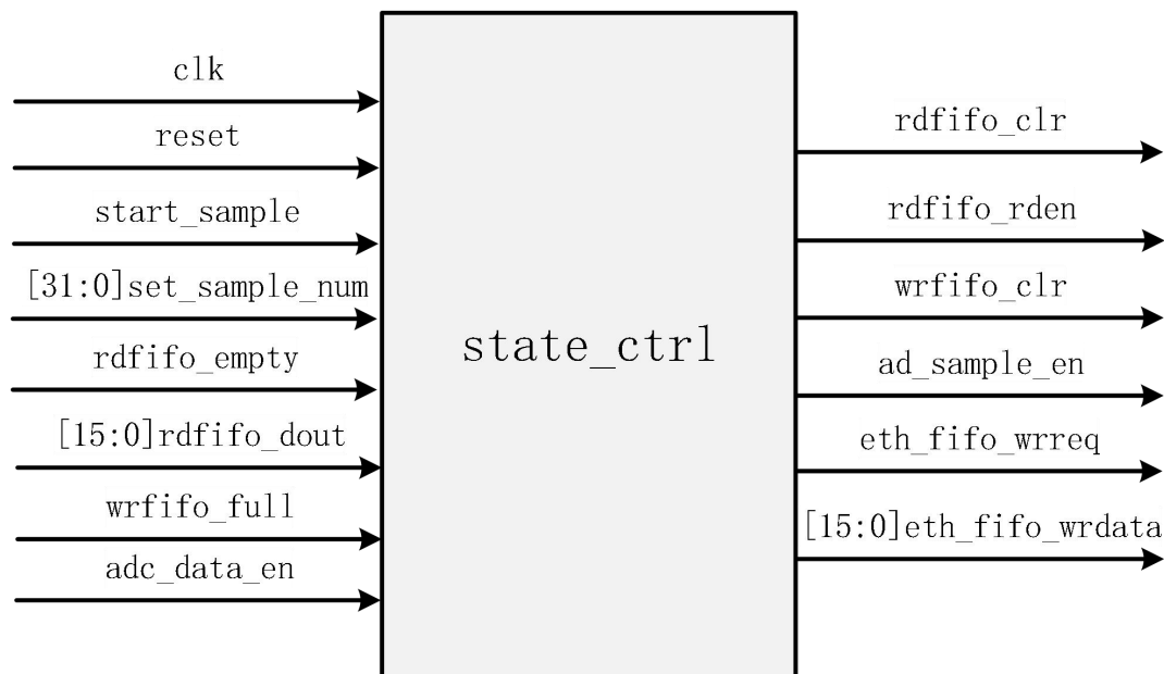
图 65-15 state_ctrl 模块结构框图
