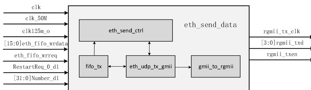
图 65-16 eth_send_data 模块基本结构框图
