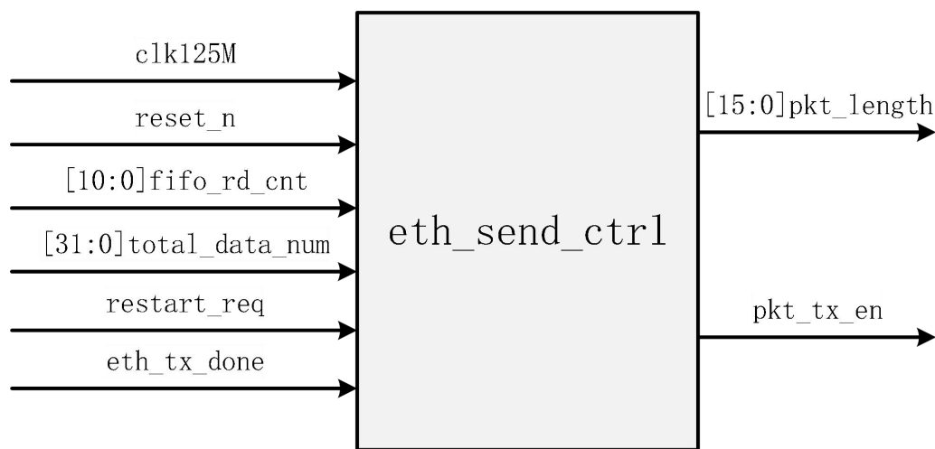
图 65-21 网口发送控制模块
