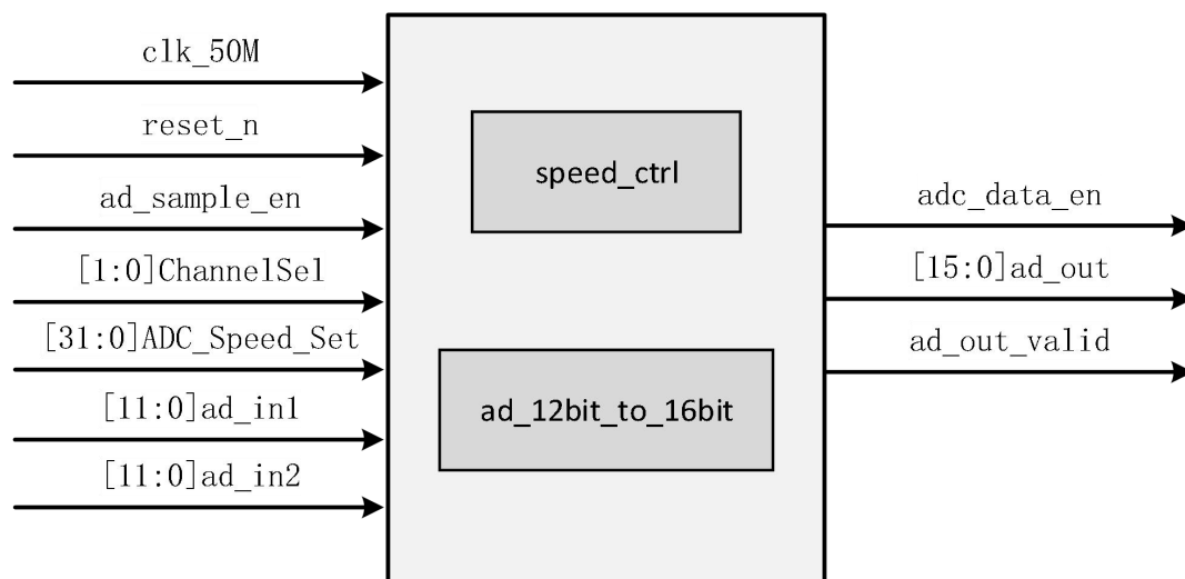
图 65-12 ad9238_ctrl 模块基本结构框图
