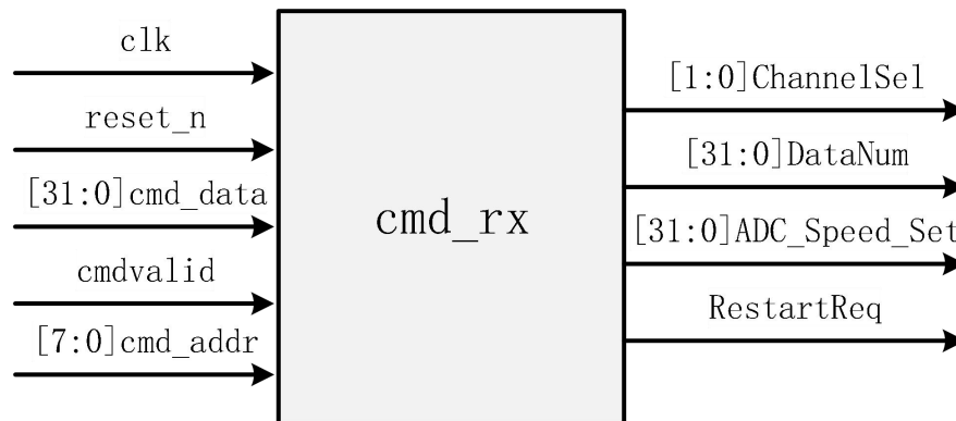
图 65-11 指令转控制模块结构框图
