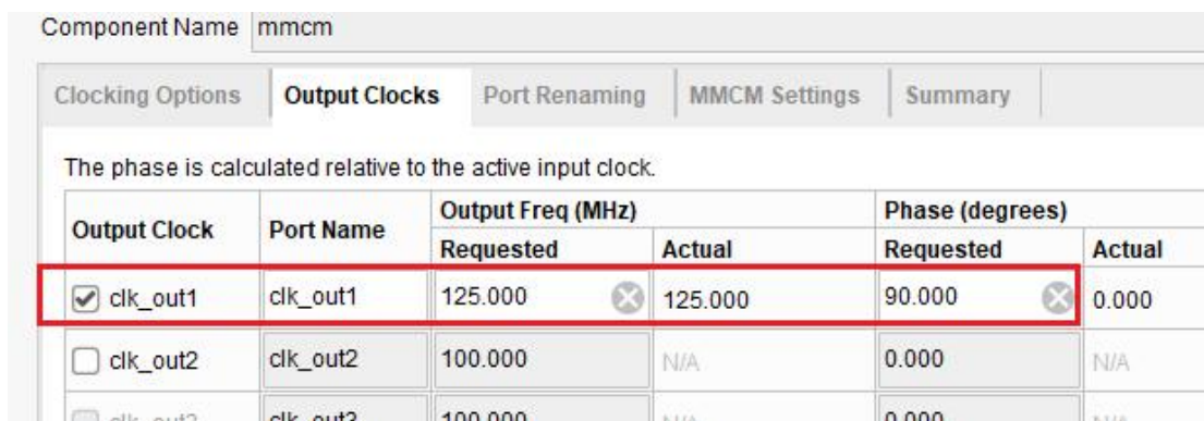
图 65-7 锁相环配置界面
