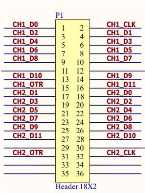
图 65-3 ACM9238 模块接口图
