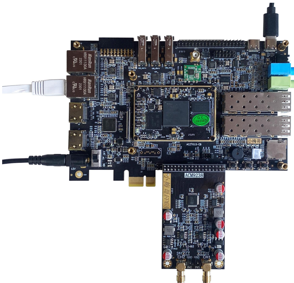
图 65-22 硬件连接图
