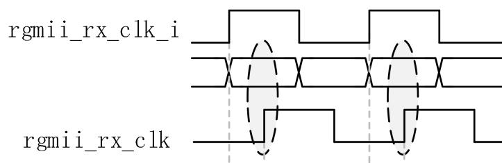
图 65-6 采集数据波形图
