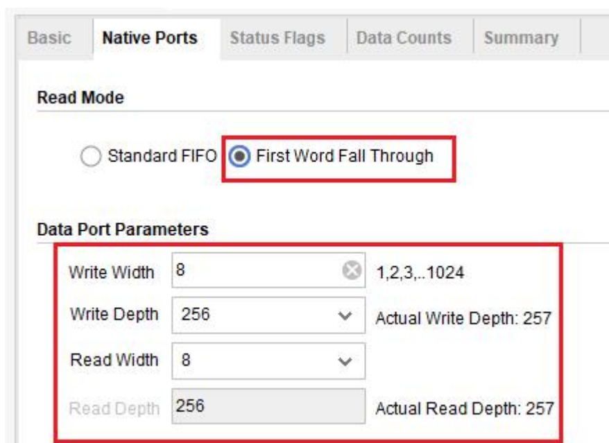
图 65-9 配置 FIFO 的读写位宽及深度
