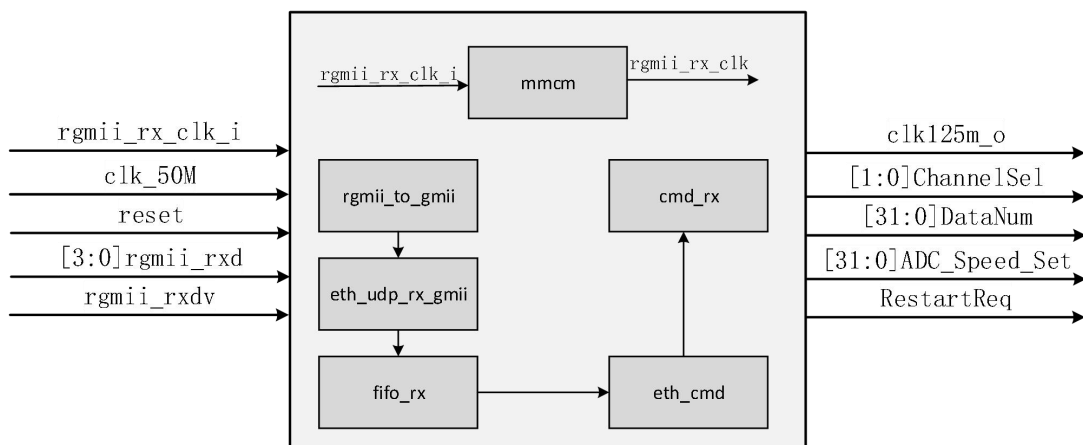
图 65-5 eth_receive_cmd 模块基本结构框图
