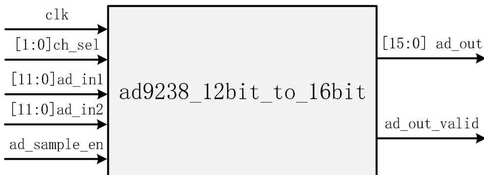
图 65-14 数据位扩展模块结构框图
