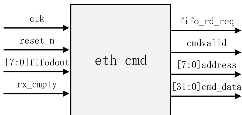
图 65-10 接收转命令模块框图
