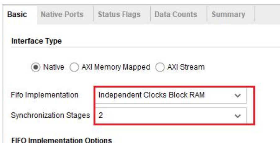
图 65-8 双端口 FIFO
