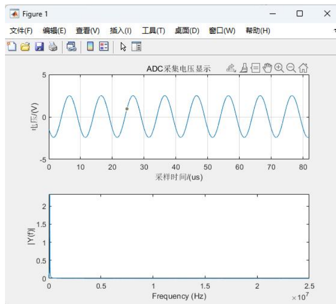
图 65-35 MATLAB 进一步波形分析图
