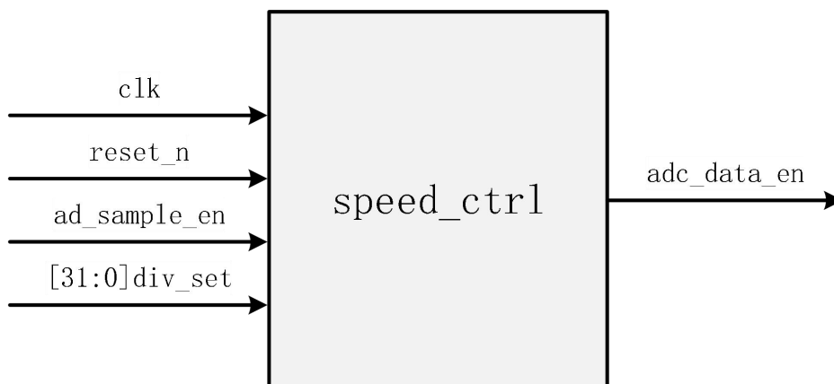
图 65-13 采样速率控制模块
