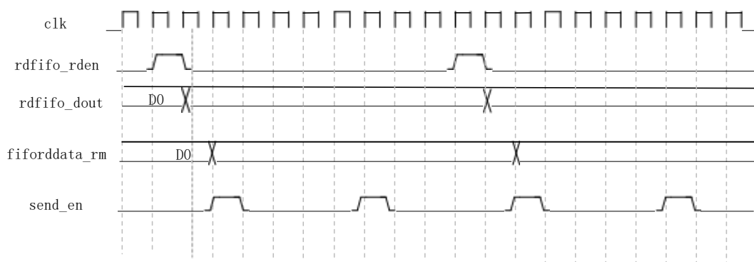
图 1-20 串口数据发送逻辑关系图
