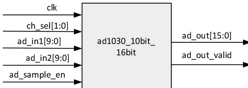
图 1-12 数据位扩展模块结构框图
