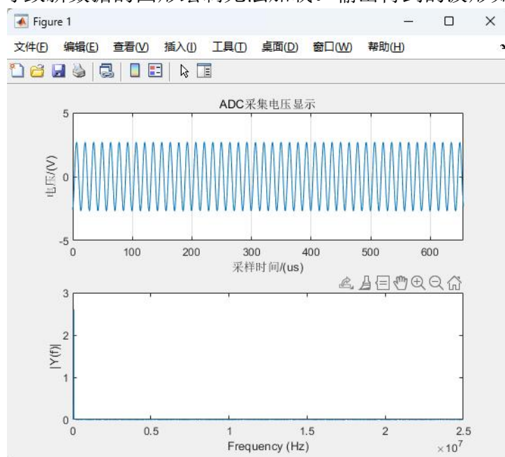
图 1-28 绘制的数据波形图
