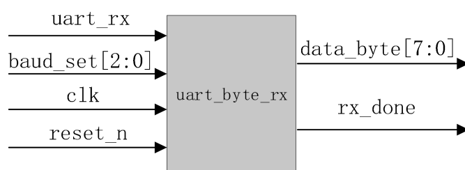
图 1-8 串口接收模块
