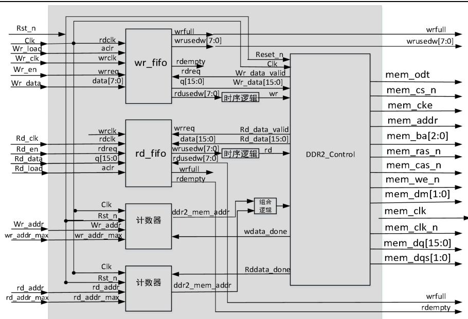
图 1-14 DDR2 控制器模块
