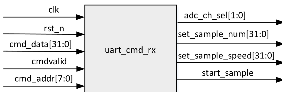
图 1-11 指令解析模块
