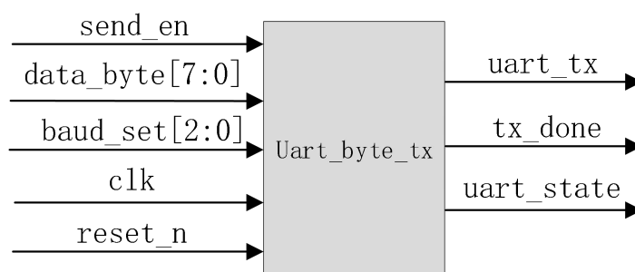
图 1-9 串口发送模块
