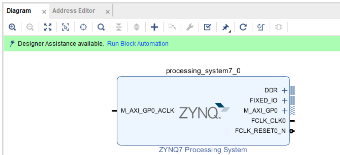
图 1-8 ZYNQ 核
