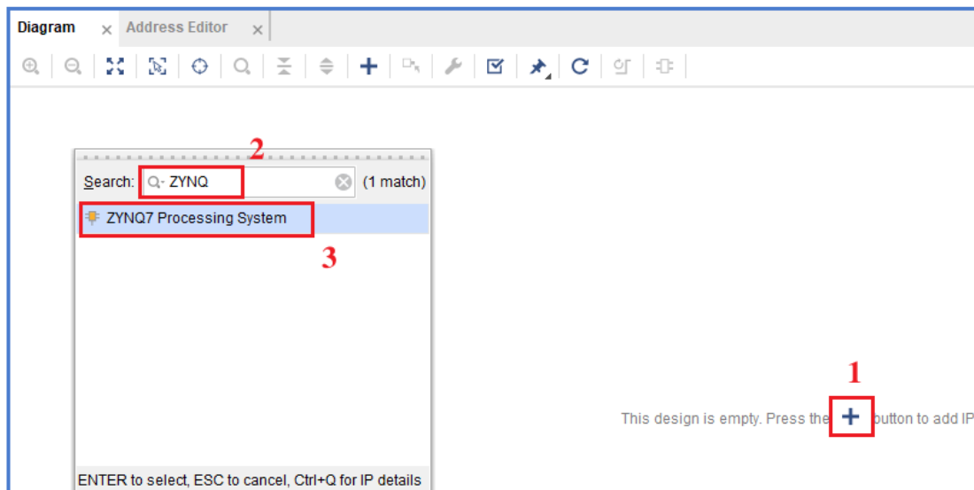
图 1-7 添加 ZYNQ 核
