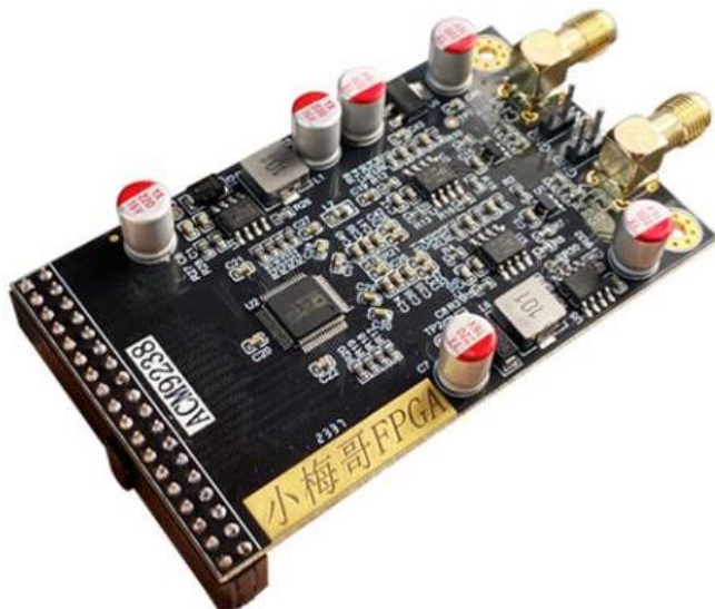
图 1-2 ACM9238 模块图
