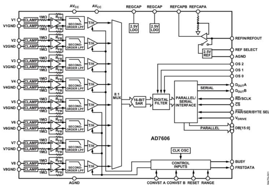
图 1-4 AD7606 功能框图
