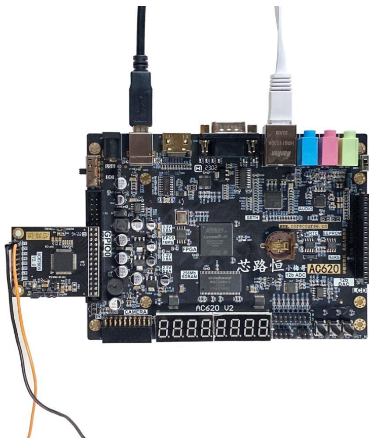
图 1-19 硬件连接图
