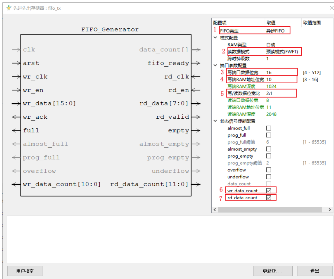
图 1-11 fifo_tx 配置界面
