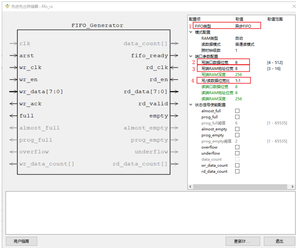
图 1-4 fifo_rx 配置界面
