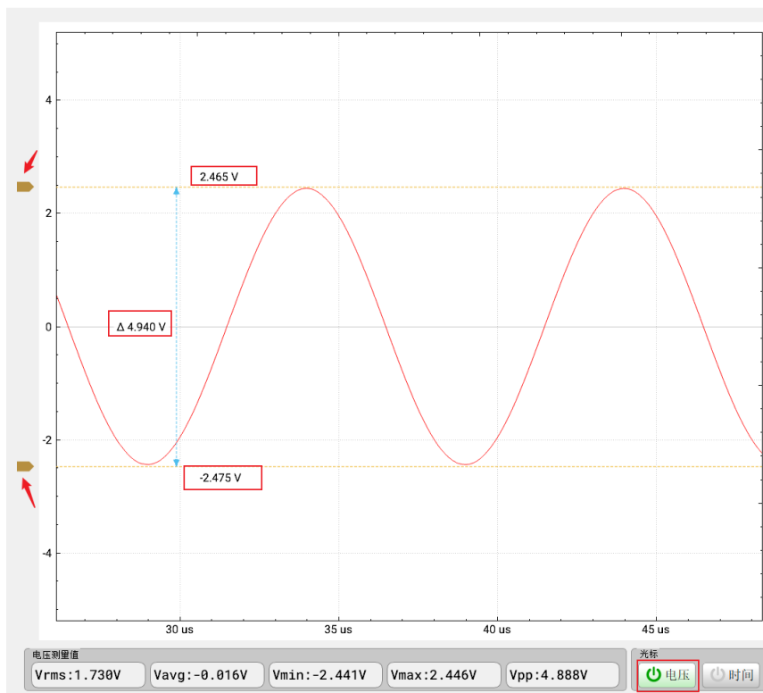
图 1-32 电压测量
