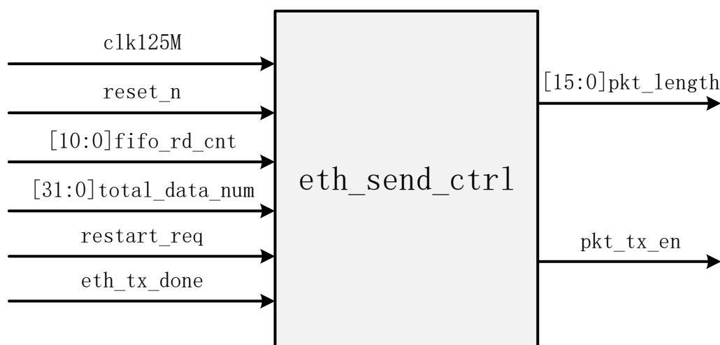
图 1-12 网口发送控制模块
